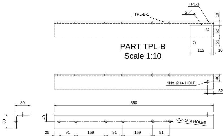
TPL-B-1 - EA 80x80x8 Scale 1:10
